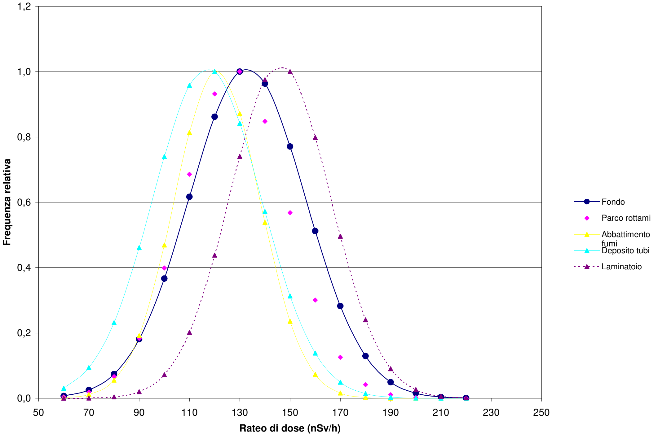
Confronto delle gaussiane dei dati con la gaussiana del fondo (normalizzati)
